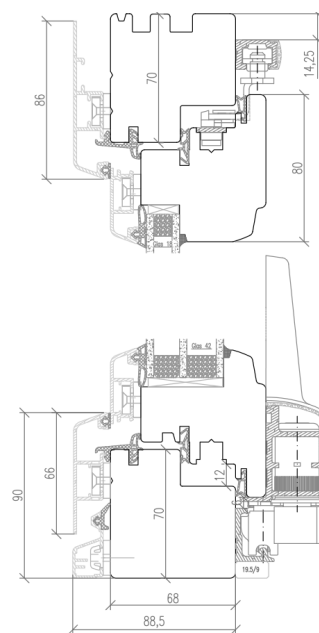
IDEALU CLASSICLINE IV 78 DETAIL HÖHENSCHNITT
