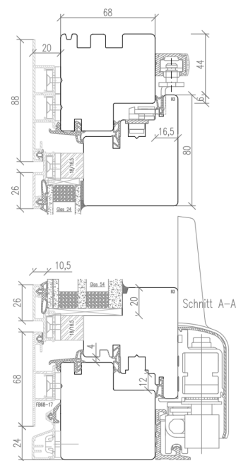
IDEAL PLANO DETAIL HÖHENSCHNITT
