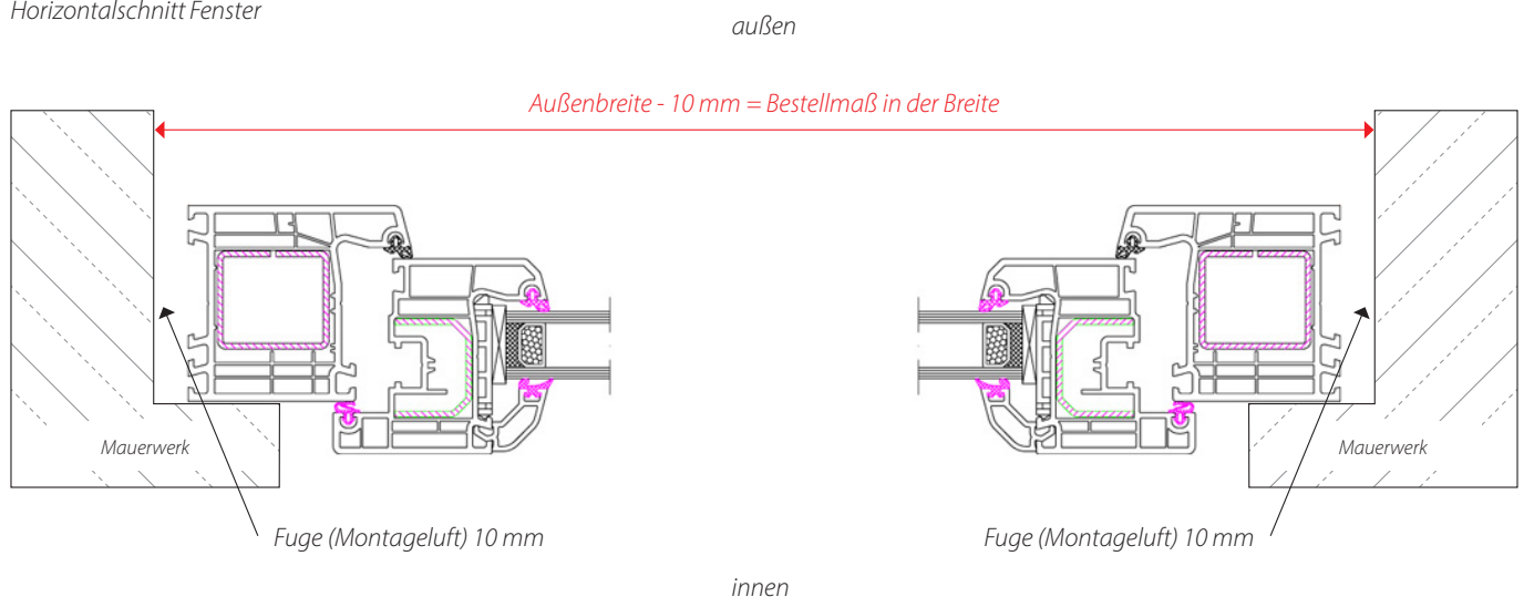
Horizontalschnitt Fenster
